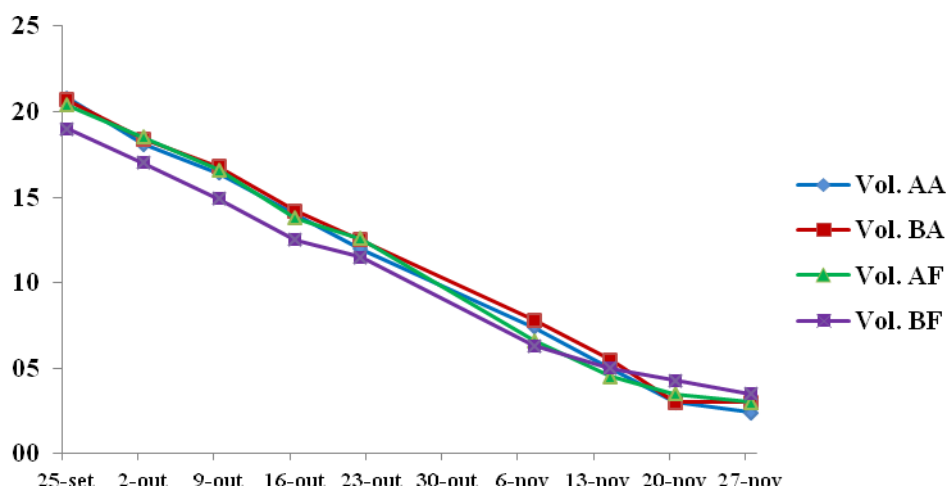
Gráfico 64 - Resultado do processo de perda de massa, dos resíduos aquosos contendo metais pesados, obtida através da evaporação passiva (2013)
